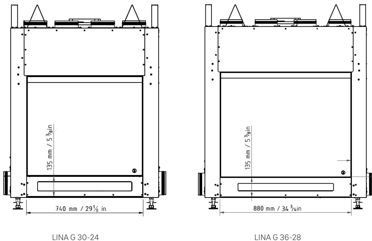
Fig.41: Panneau d'accès
